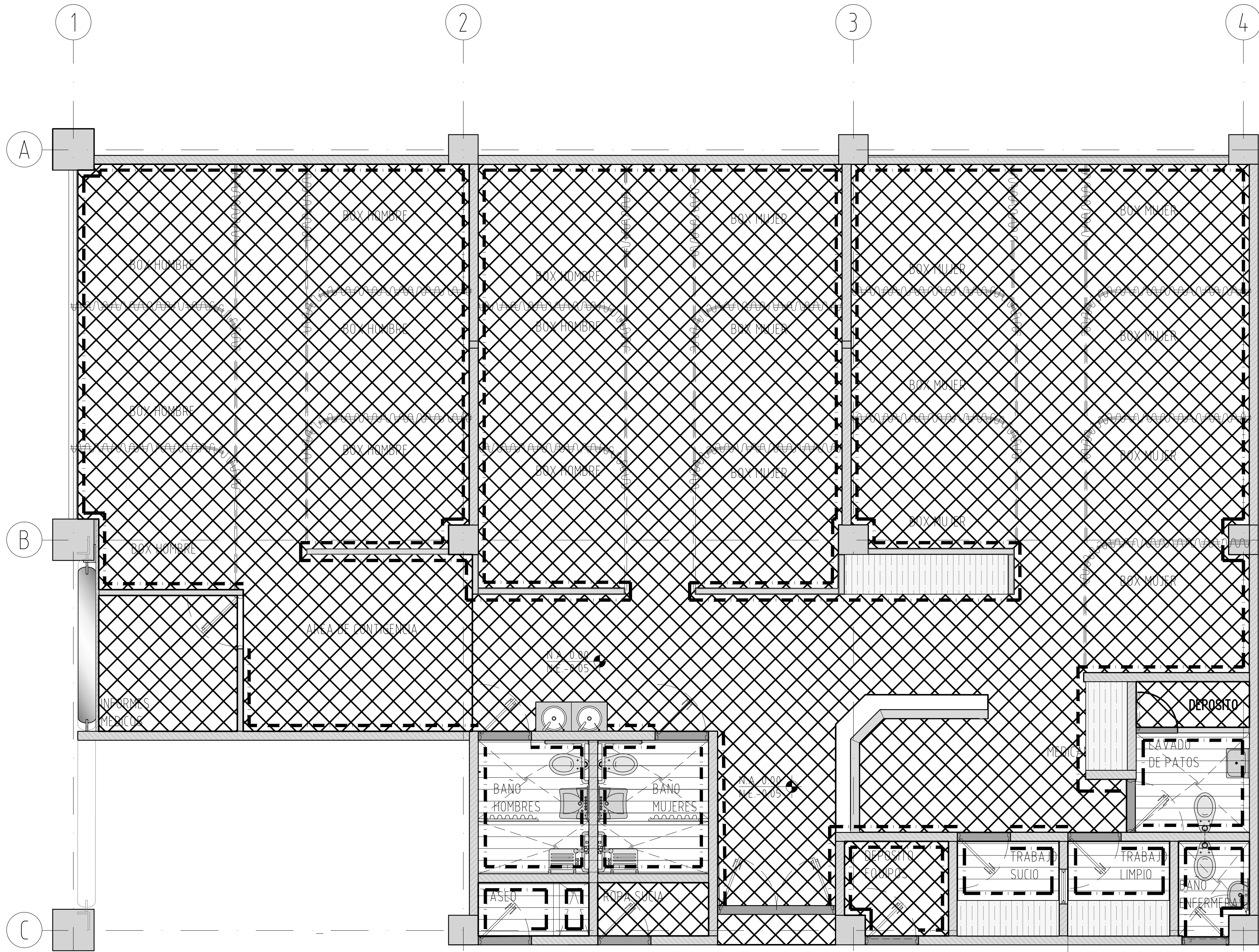
PLANTA TIPO DE PISOS ESC:130
