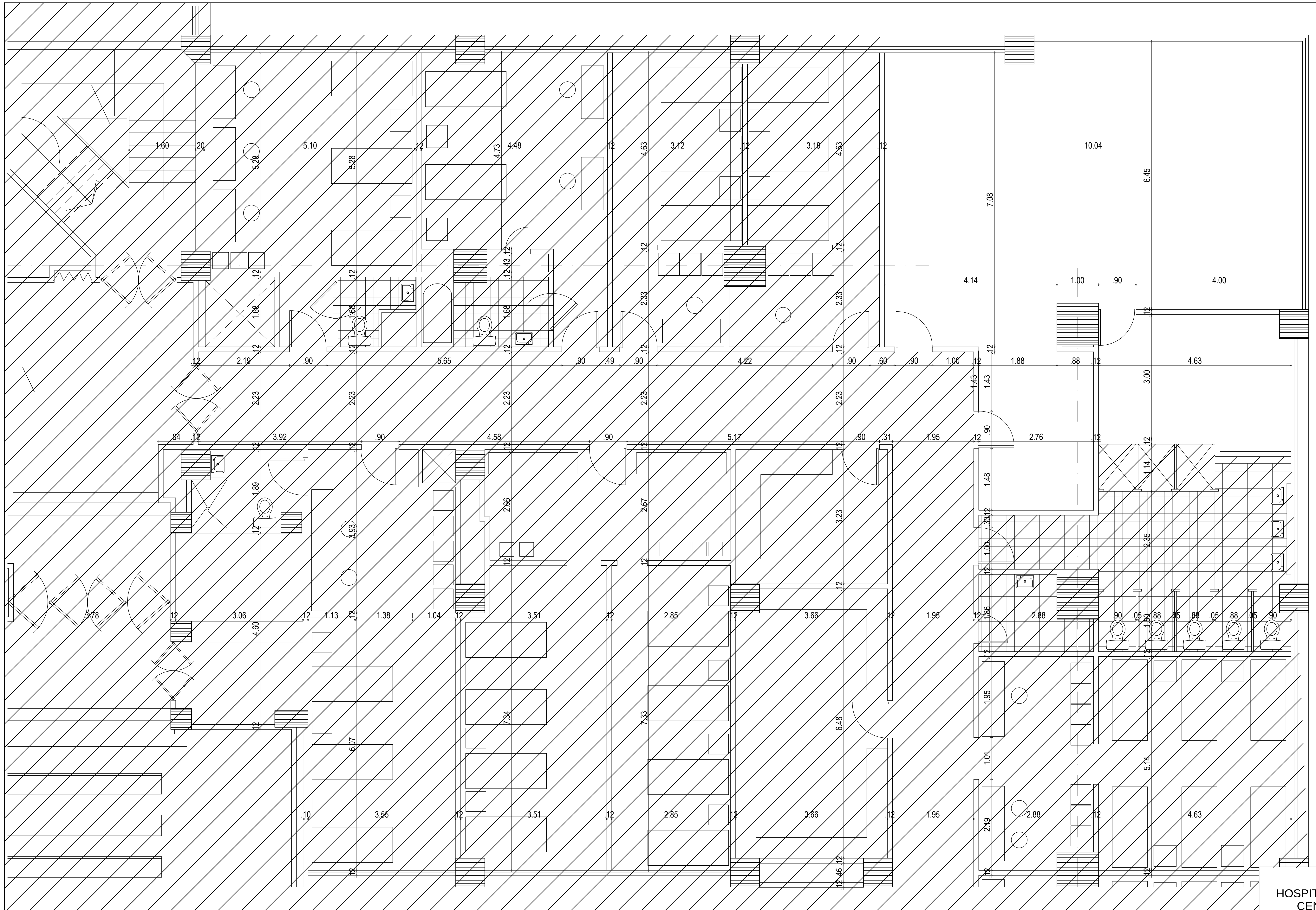
AREA DEL CLUB MEDICO SOTANO 1
